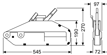
Yaletrac Y16
