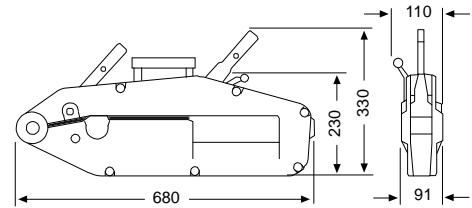
Yaletrac Y32
