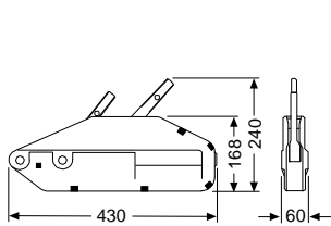
Yaletrac Y08
